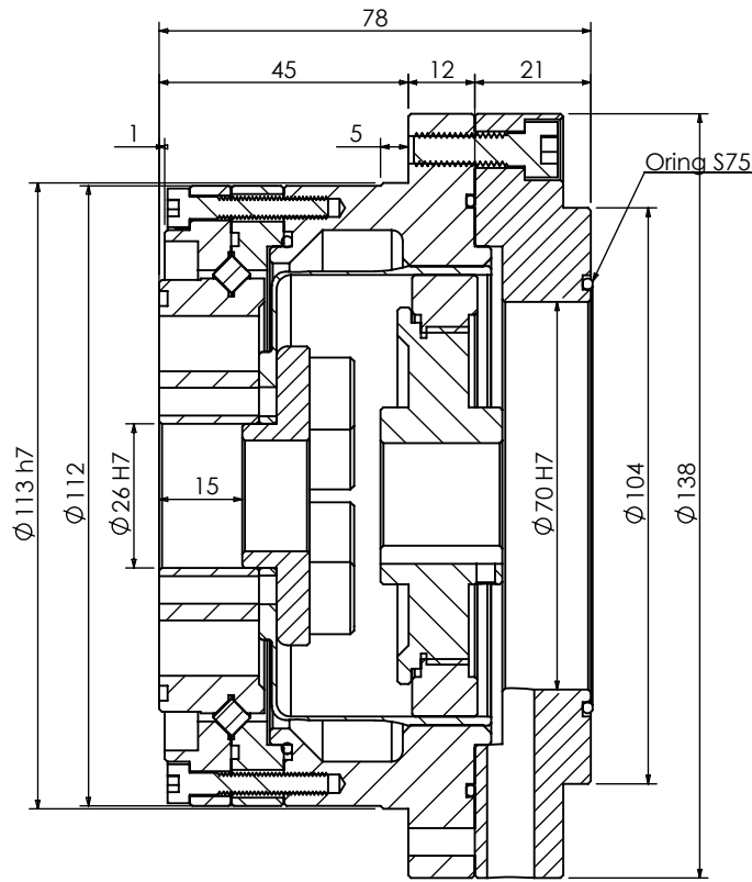
CT-CT (1 : 1.5)
